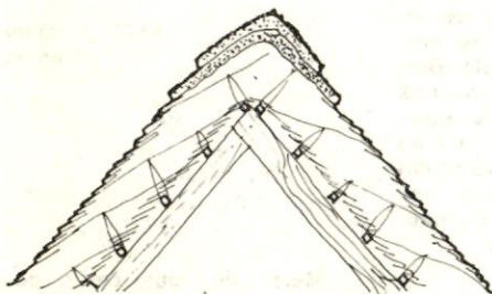
faitage en mottes de gazon
