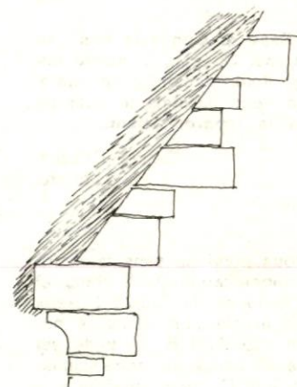
chevronnières
