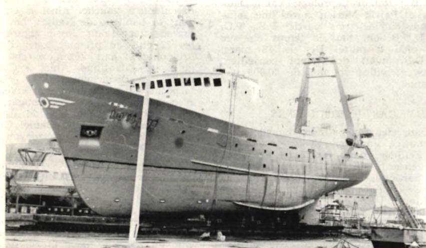
Chalutier en construction aux chantiers la Perrière.
