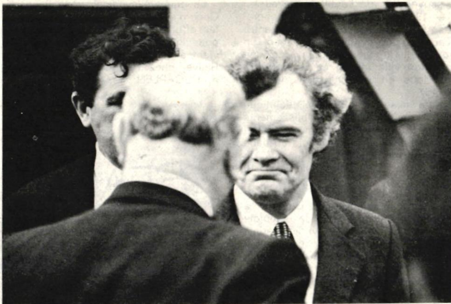
Guermeur (R.P.R.)
